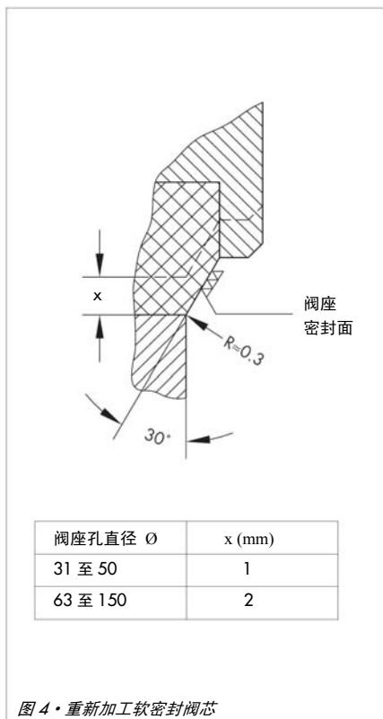
图 4 • 重新加工软密封阀芯
